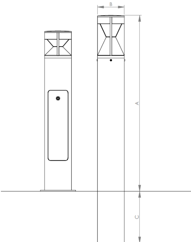
Fig. 1 - Pharola Max Range
